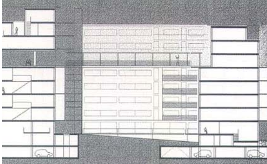
Querschnitt
