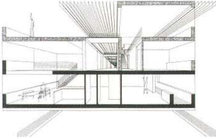
Schnittperspektive „Flieger“
