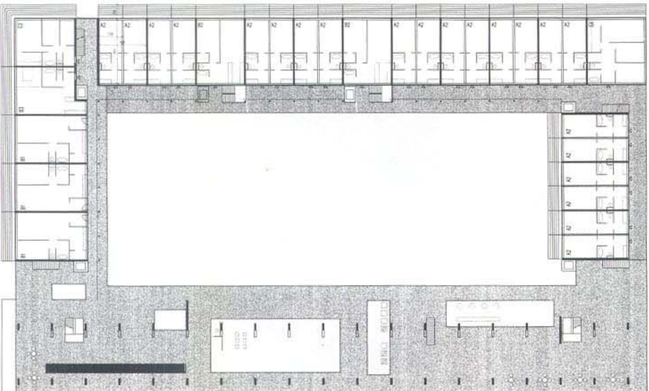
5. OG: Aussichts- und Sozialgeschoß
