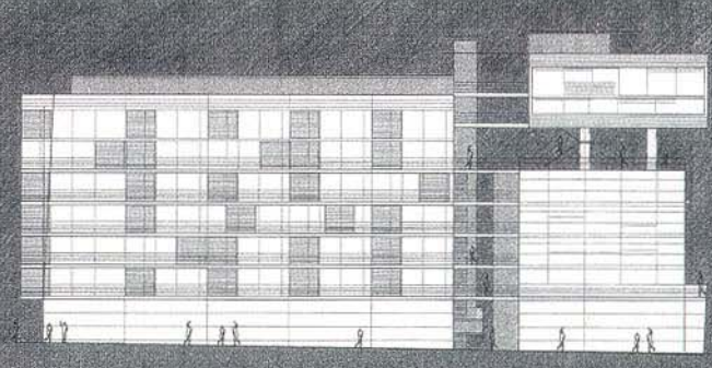
Ansicht Machstraße
