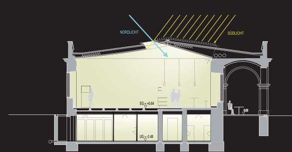
SCHNITT B
