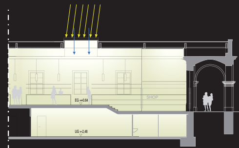
SCHNITT A
